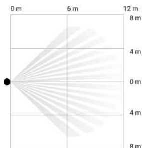
Angle de vue horizontal du détecteur
