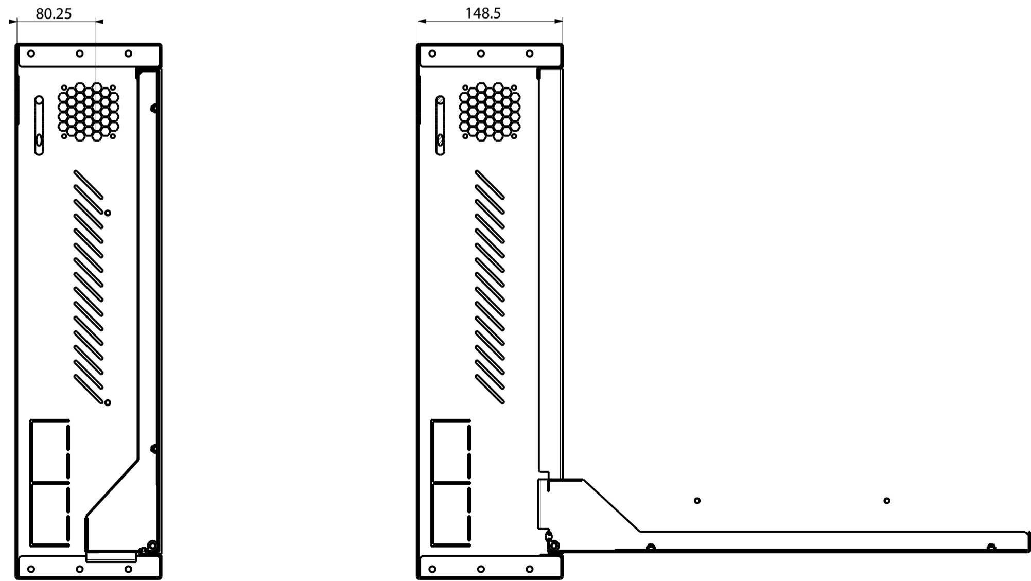
SEZIONE A-A
