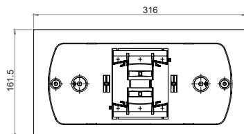
Cadre d'encastrement (mm)
