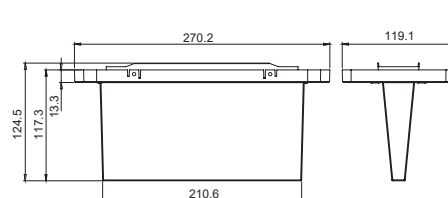
Kit signalétique plafond (mm)
