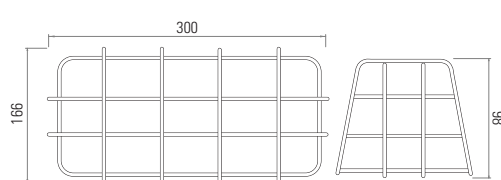
Grille de protection (mm)
