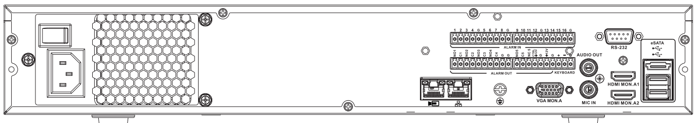
Panneau arrière DIVAR 5000 network (non PoE)
