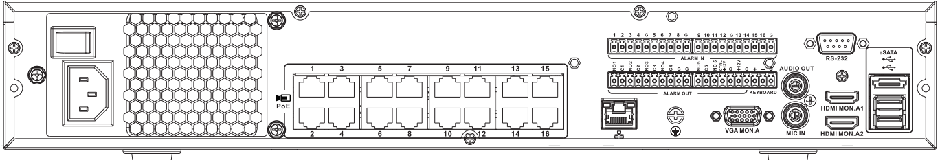
Panneau arrière DIVAR 5000 network (16 PoE)
